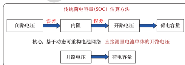
图2 基于可重构电池网络SOC估计原理
