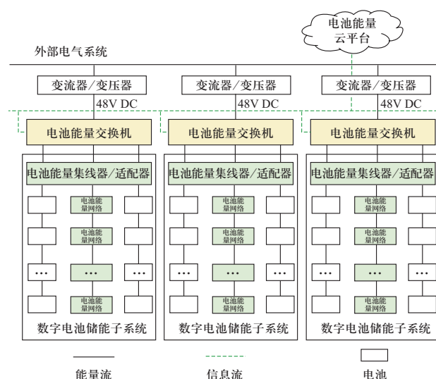
图5 系统整体架构图
