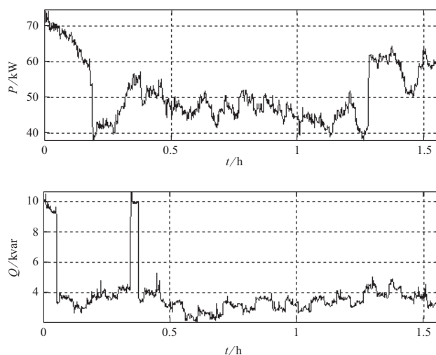
图10 单相基波功率趋势
