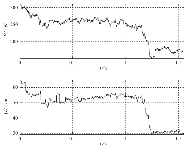
图9 总线基波功率
