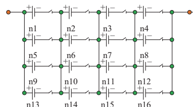
图1 可重构电池网络设计 [13]
